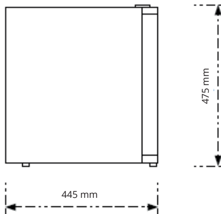
zij-aanzicht
