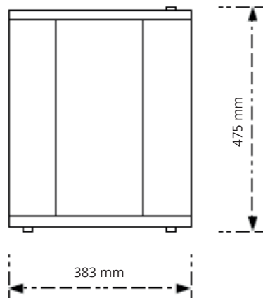
vooraanzicht
