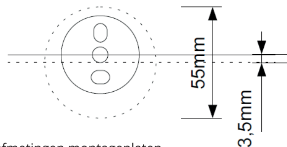
afmetingen montageplaten
