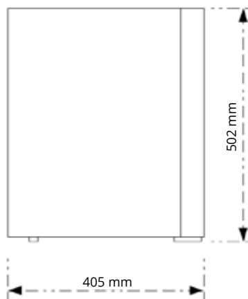
zij-aanzicht
